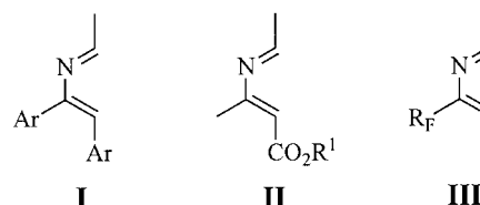
Figure 1. 2-Aza-1,3-butadienes I–III .
